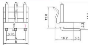
HX39603-WAG (5274/3.96)
