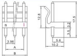
HX39603-A (5273/3.96)
