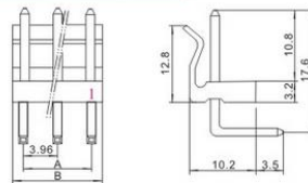
HX39603-WAG (5274/3.96)
