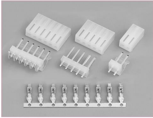
端子 TERMINAL(4018/3.96)
