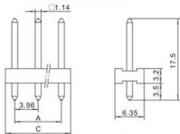
HX39603-A (5273/3.96)
